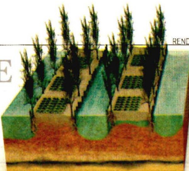
RENDER 3D: OSCAR CASTRO ESTRUCTURA DE UNA CHINAMPA.
